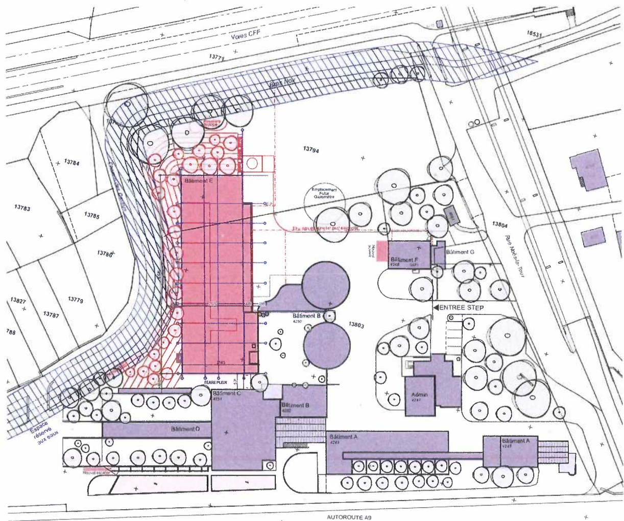
Figure 7 : Vue sur le nouveau bâtiment E pour le traitement de l'azote et des micropolluants.
